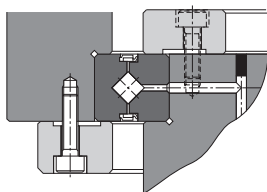
RE型 安装例
