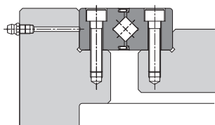
图3 RU型 安装例
