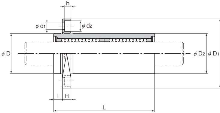
LMIH-L型
