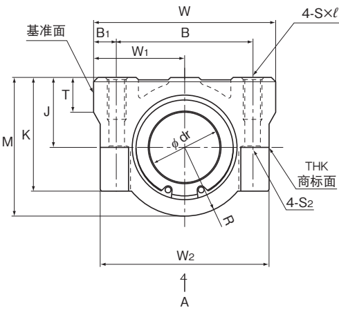
SC35~50型
