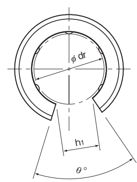
LME-OP型
