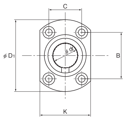
LMIH 16L~25L型
