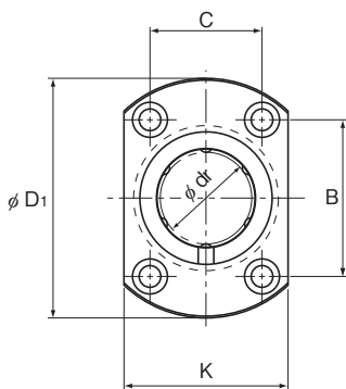
LMH16~30型
