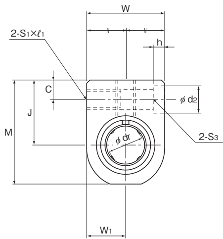
SH-L型
