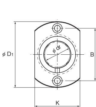
LMH 6~13型
