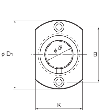
LMH 6M~13M型
