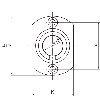
LMIH 6L~13L型
