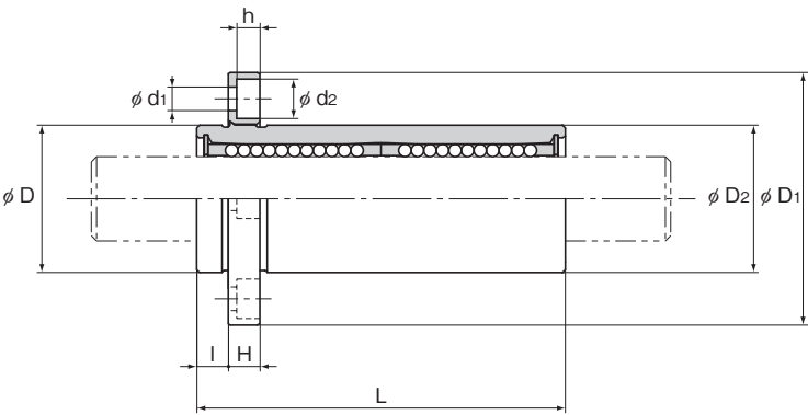
LMIF-L型
