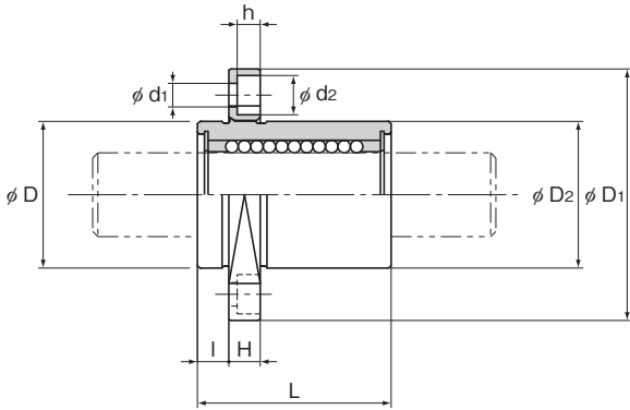
LMIH型
