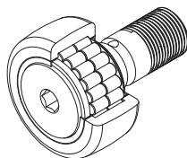
NUCF-AB型
